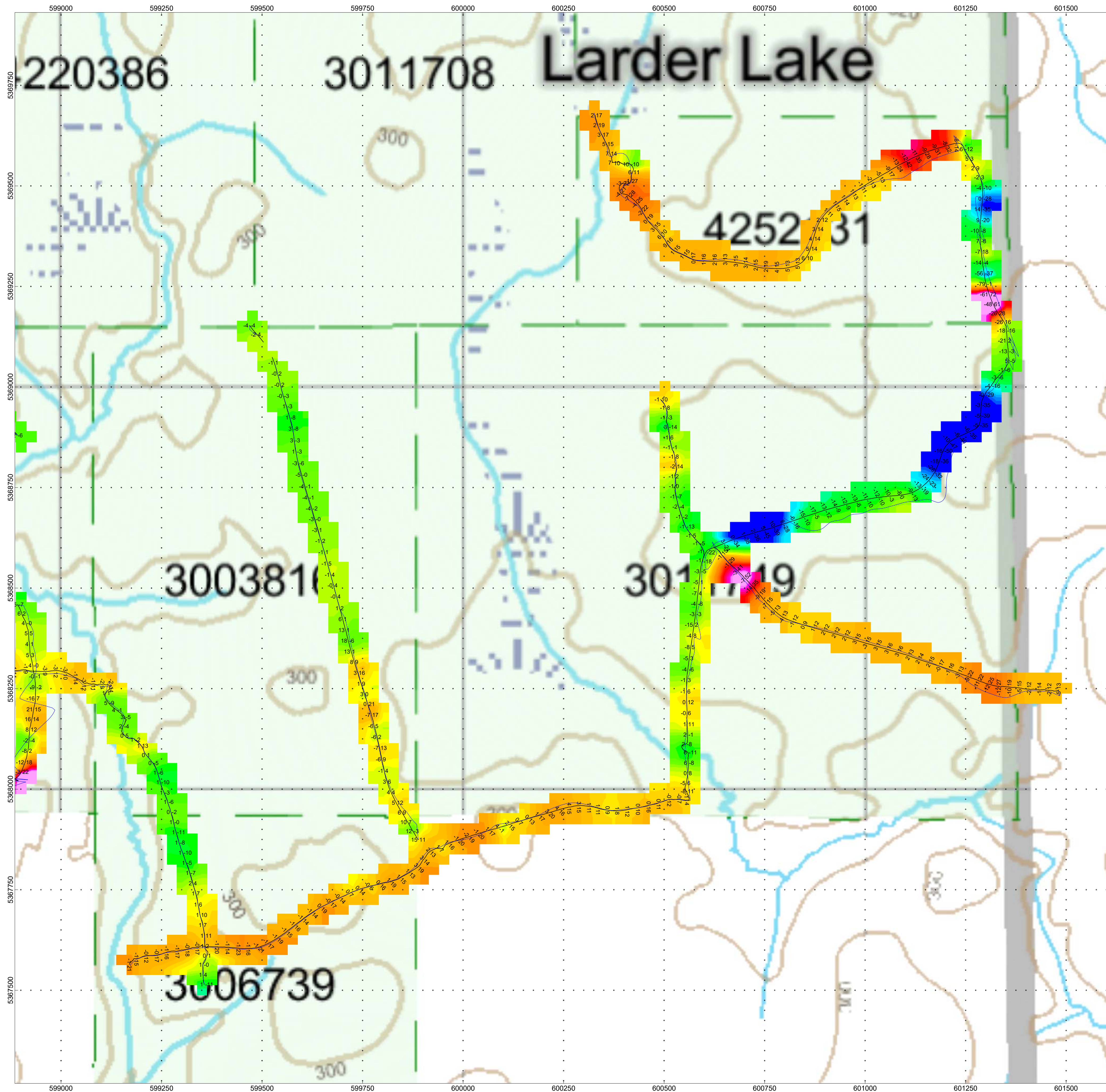
VLF EM IN-PHASE percent
